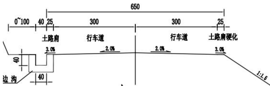
图 2.1-1 路基标准横断面图
