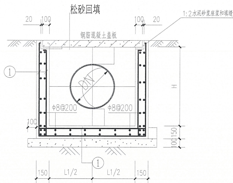
车行道管沟详图
