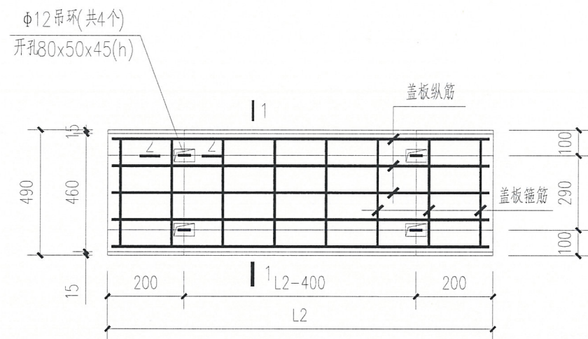
盖板详图
