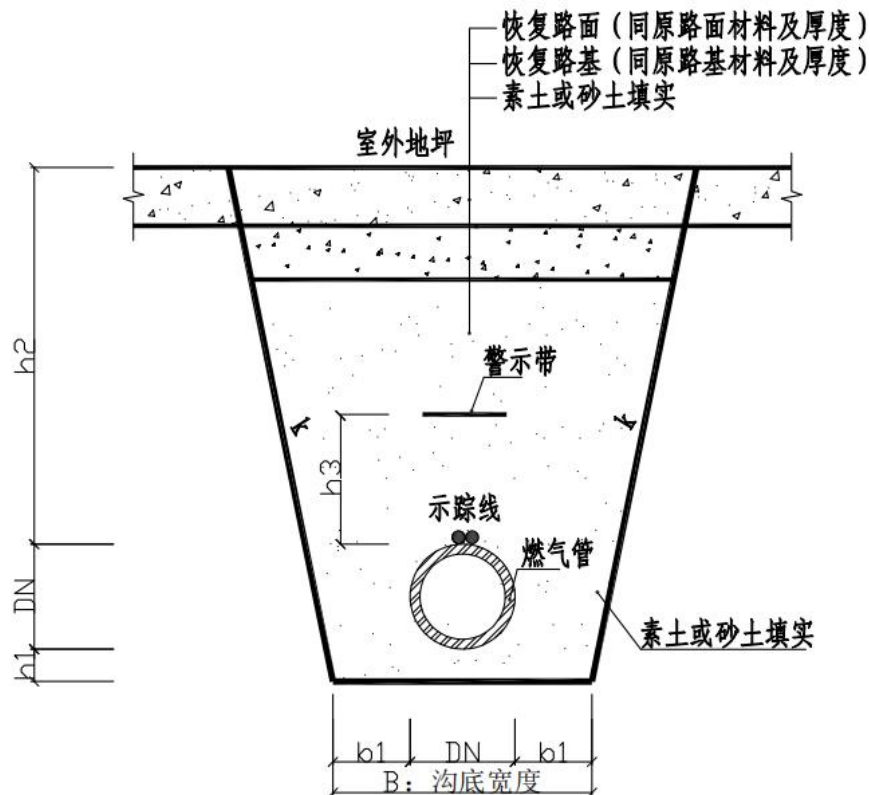
图 2.1-2 管道开挖断面图
