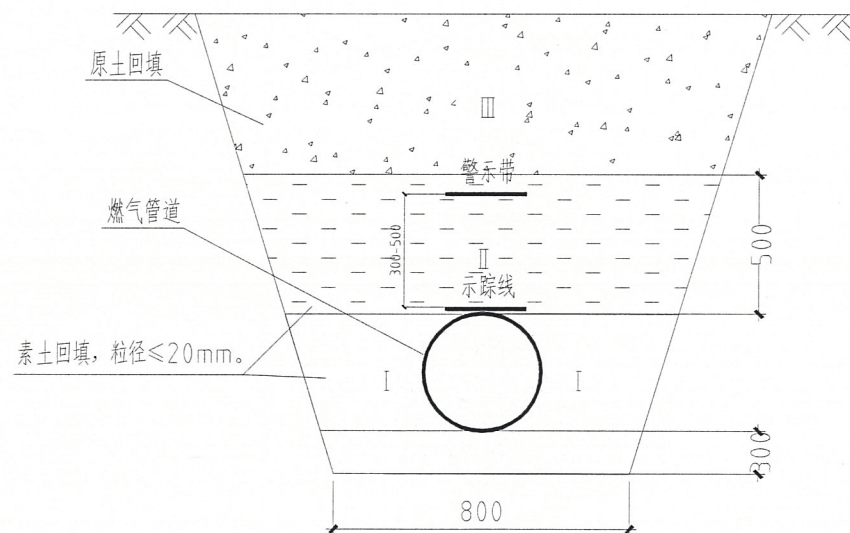
一般段管沟槽断面图
