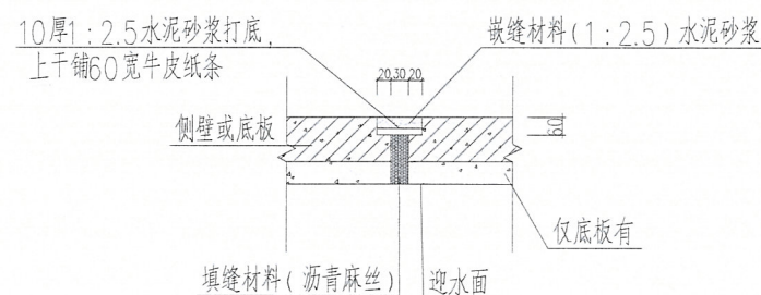
变形缝大样
