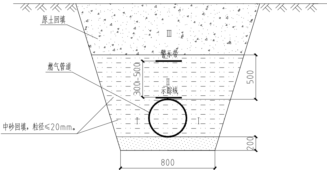
一般段管沟槽断面图
