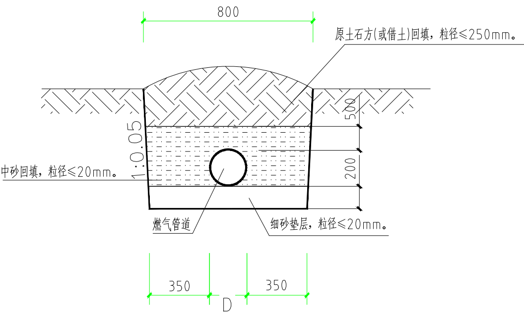
硬质岩管沟槽断面图
