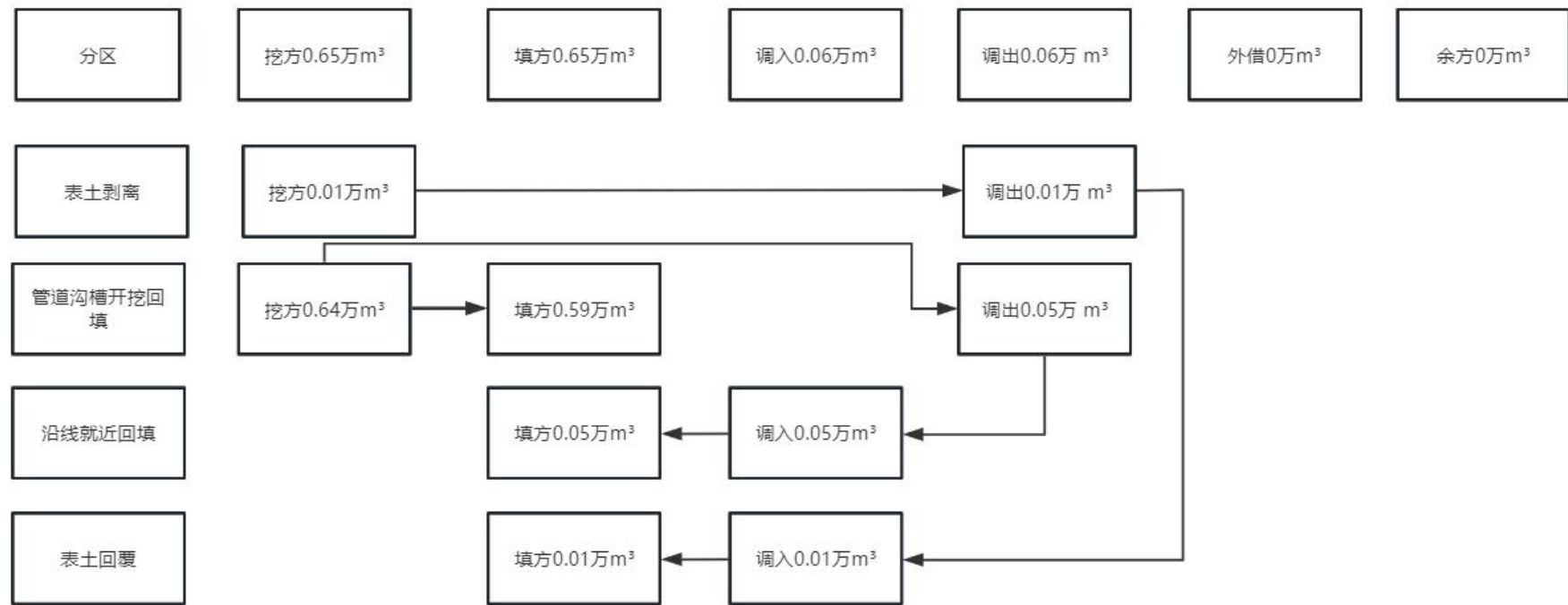
图 2.4-1 土石方流向框图 (单位: 万 m³)
