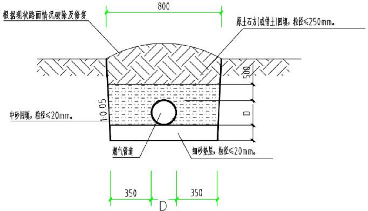
图 2.1-3 管道开挖断面图（二）
