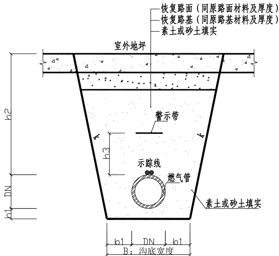
单管沟断面图
